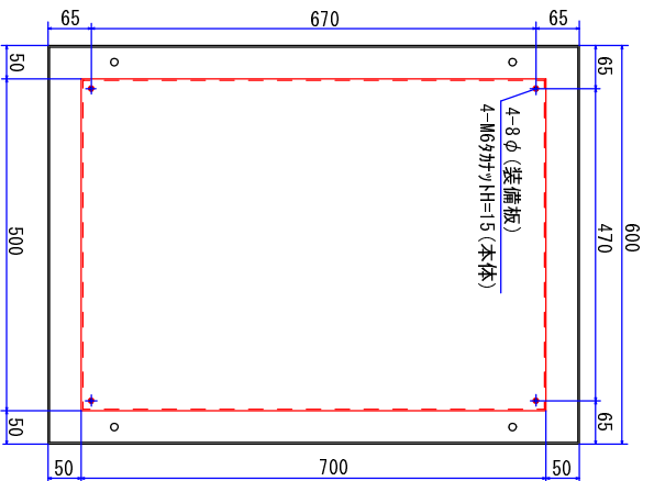
A-B矢視
