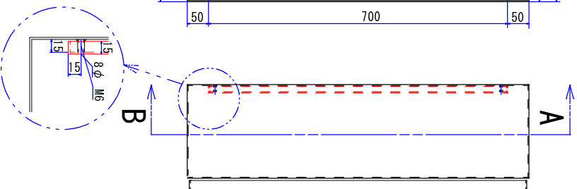
左側面図
