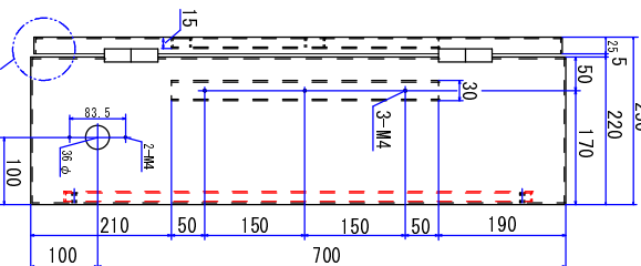
右側面図
