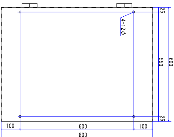
背面図
